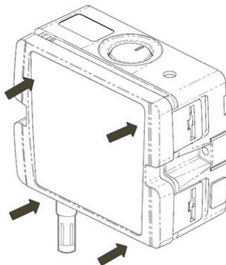
Figura 20 – Encaixe da tampa do dispositivo
