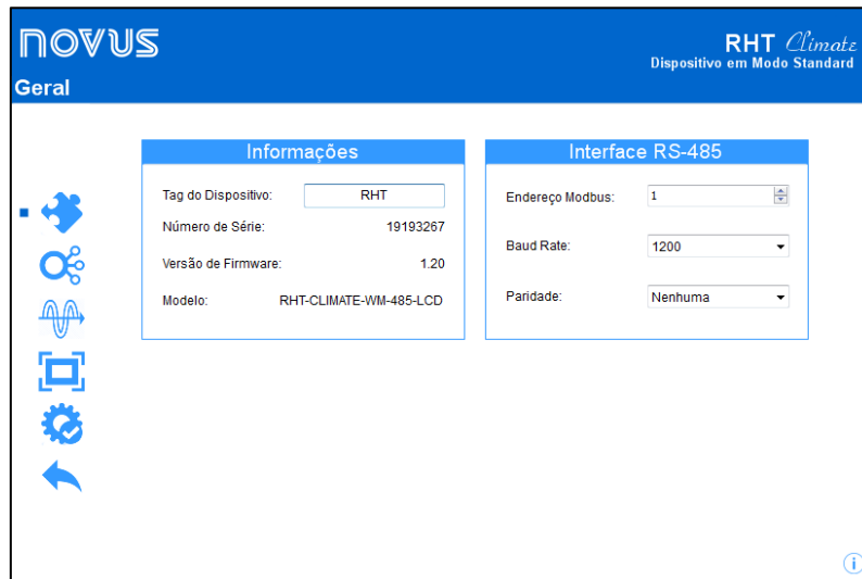
Figura 30 – Tela de configuração
