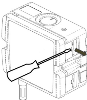
Figura 18 – Retirando a tampa do dispositivo (1)
