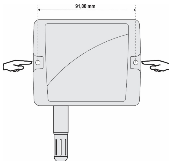
Figura 14 – Instalação Mecânica
