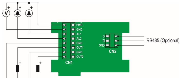
Figura 21 – Conexões elétricas
