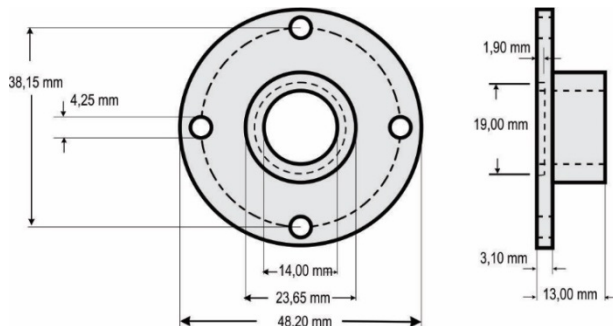
Figura 16 – Flange para a fixação do modelo DM
