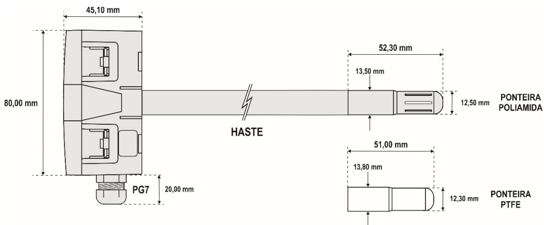
Figura 17 – Dimensões do modelo DM
