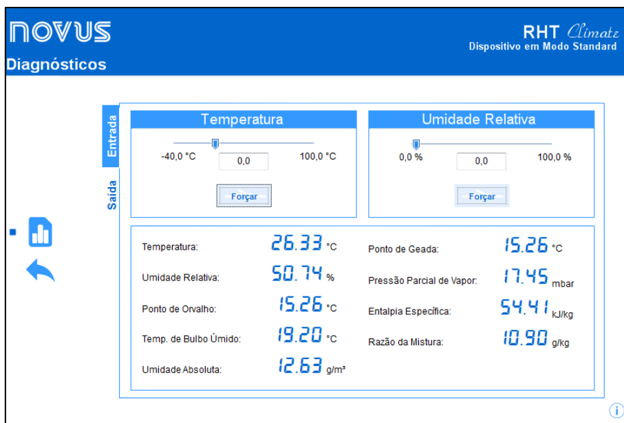
Figura 42 – Tela de diagnósticos de entrada (1)
