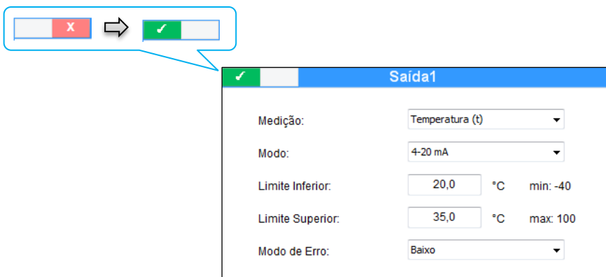
Figura 34 – Tela de configuração da saída 1
