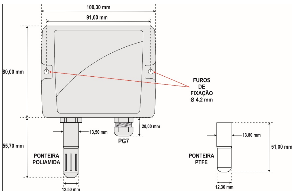
Figura 15 – Dimensões do modelo WM
