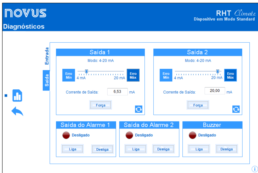
Figura 44 – Tela de diagnósticos de saída
